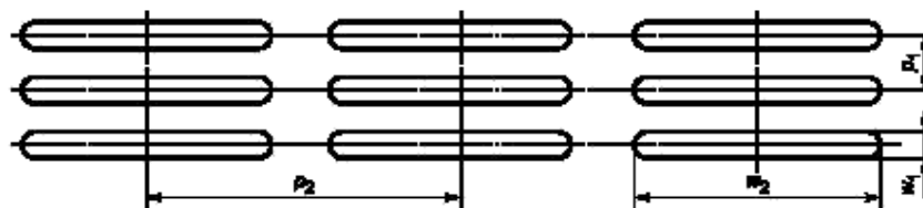
Рисунок 1 — Лабораторные сита с продолговатыми округленными отверстиями
