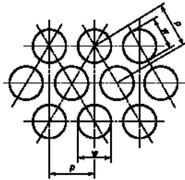
Рисунок 2 — Лабораторные сита с круглыми отверстиями
